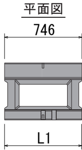
5分用基礎Ⅱ型
