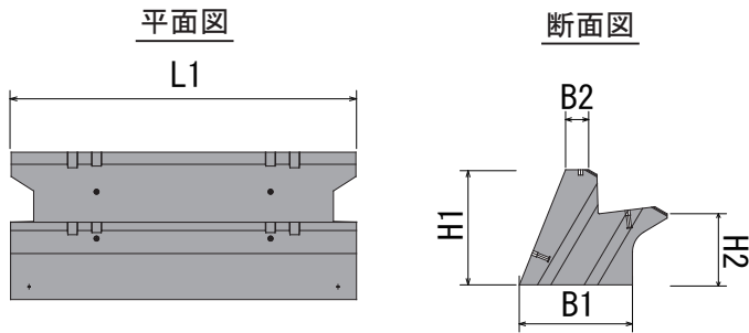
1割5分用基礎
