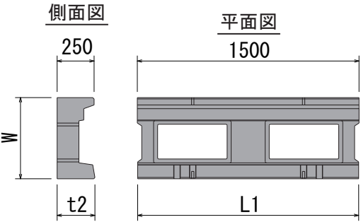
3分・4分用基礎Ⅰ型
