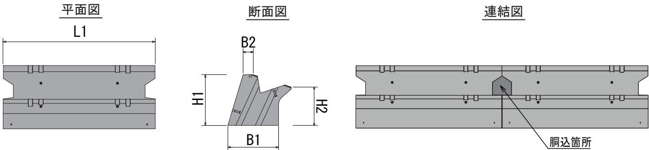
1割用基礎
